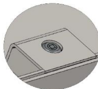
Detail verrouillage
